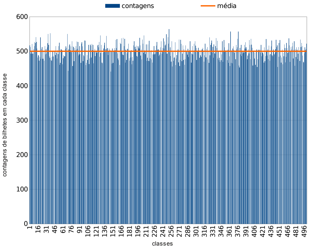
Figura 1: Histograma de Bilhetes Premiados
